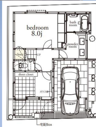
1階平面図
