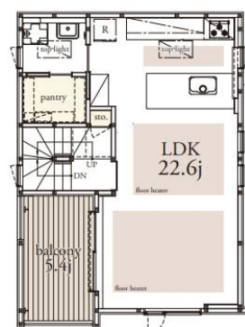
2階平面図
